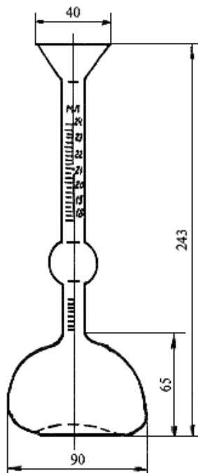
Рисунок 8 - Прибор Ле Шателье
