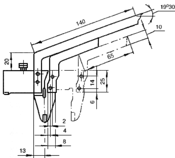
Рисунок 3 - Передвижной шаблон
