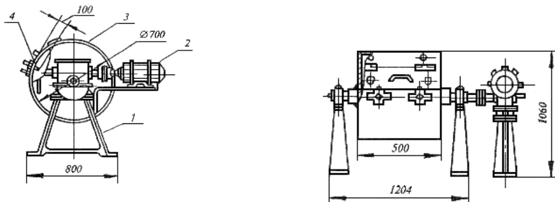
1 - станина; 2 - двигатель; 3 - барабан; 4 - полка барабана
